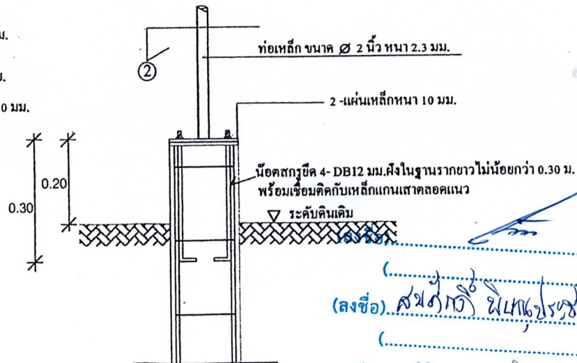
แบบขยายค่อม่อ 2 NOT TO SCALE
