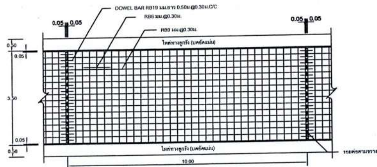
แปลนแสดงการเสริมเหล็กถนน คสส. NOT TO SCALE
