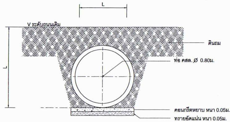
รูปตัดท่อระบายน้ำ คสล. \varnothing 0.80ม. ยาว 1.00ม.
