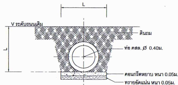
รูปตัดท่อระบายน้ำ คสล. \varnothing 0.40ม. ยาว 1.00ม.
