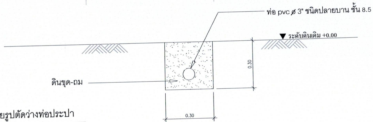
แบบขยายวางท่อประปา มาตราส่วน No Scale
