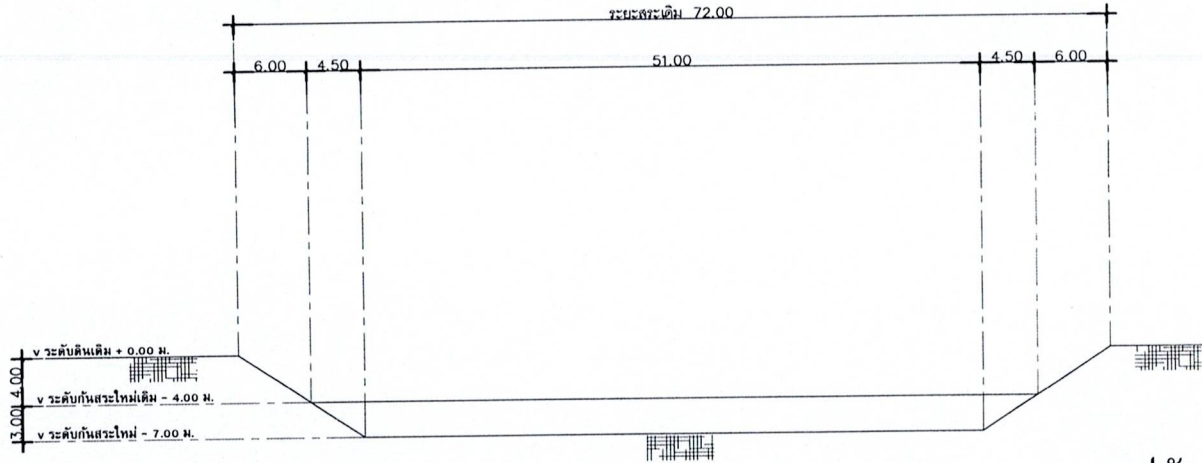
รูปตัด B SCALE NO
