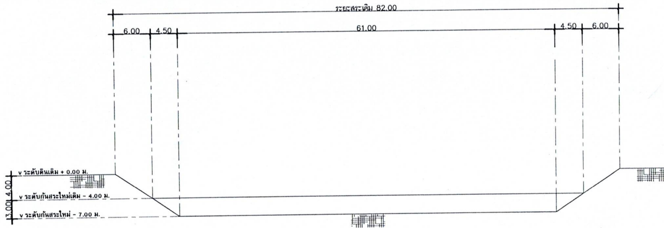
รูปตัด A SCALE NO
