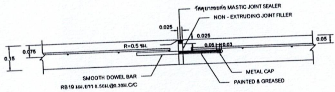
ขยายข้อต่อ EXPANSION JOINT NOT TO SCALE
