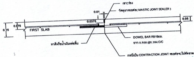
ขยายข้อต่อ CONSTRUCTION JOINT และ CONTRACTION JOINT NOT TO SCALE
