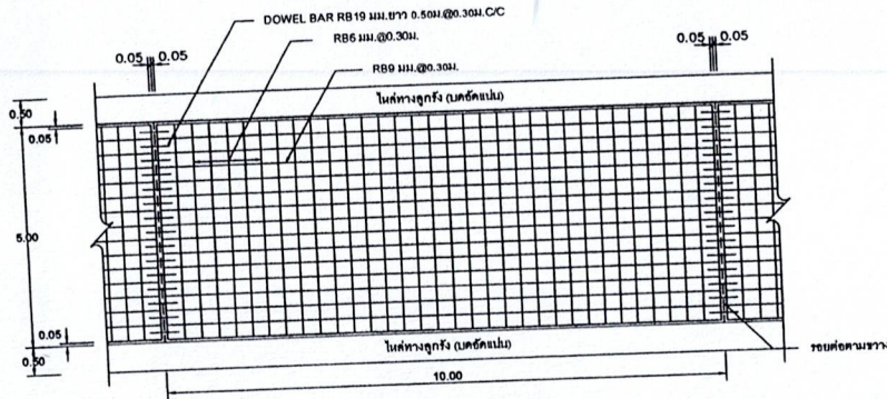
แปลนแสดงการเสริมเหล็กตาม คคค. NOT TO SCALE
