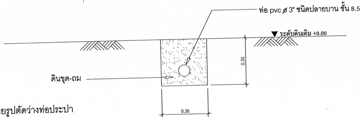
แบบขยายวางท่อประปา มาตรฐาน No Scale
